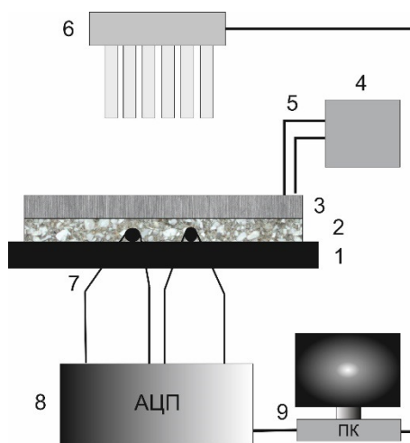
Рис.1. Схема экспериментальной установки. 1 – подложка, 2 – смесь PbO 2 + В с добавкой Al 2 O 3 и порошка стекла, 3 – смесь Ni + Al, 4 – генератор, 5 – поджигающие электроды, 6 – оптический сенсор, 7 – термопары, 8 – АЦП, 9 – персональный компьютер.
